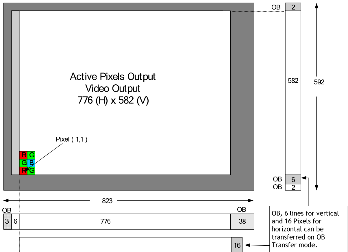
Fig. 17. CCD sensor layout
