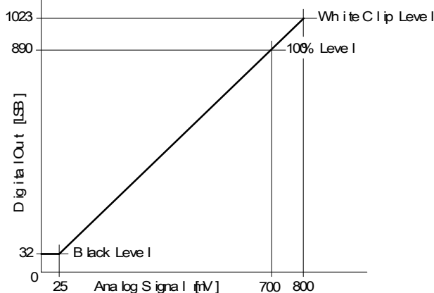
Fig. 10. Digital Output
