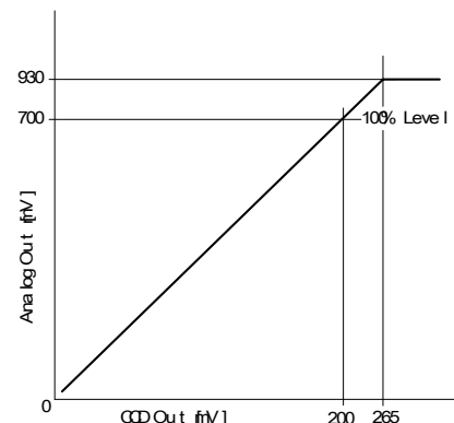
Fig. 14. Iris video output.
