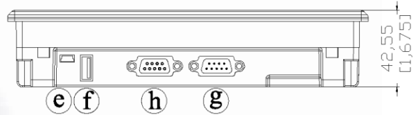
底视图
