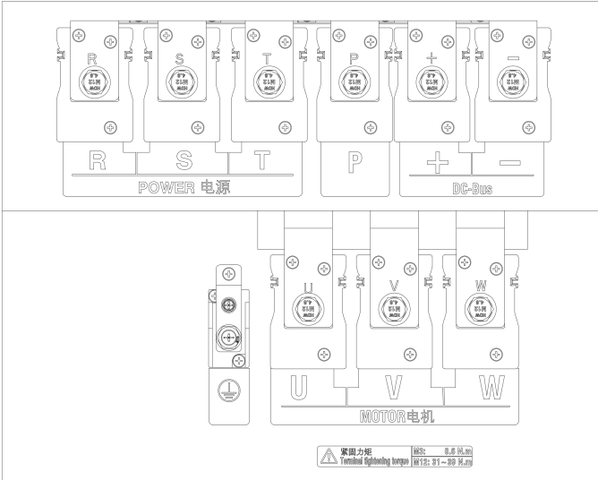
(f) EM730-132-3~EM730-160-3 端子示意图
