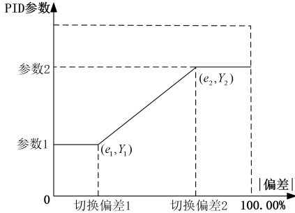
图 9- 28 PID 参数根据偏差自动切换 (F19.11=2) 示意图
