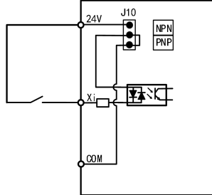
b: PNP 模式使用内部电源
