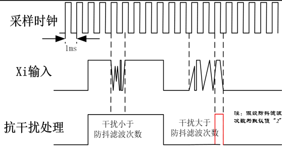
图 7- 13 端子滤波采样示意图
