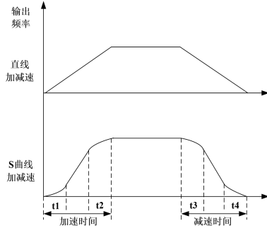
图 7- 16 加减速时间控制图
