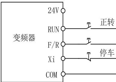
(a) F00.03=2 三线控制接线示意图
