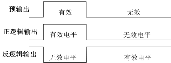
图 7- 14 数字输出端子正反逻辑输出示意图
