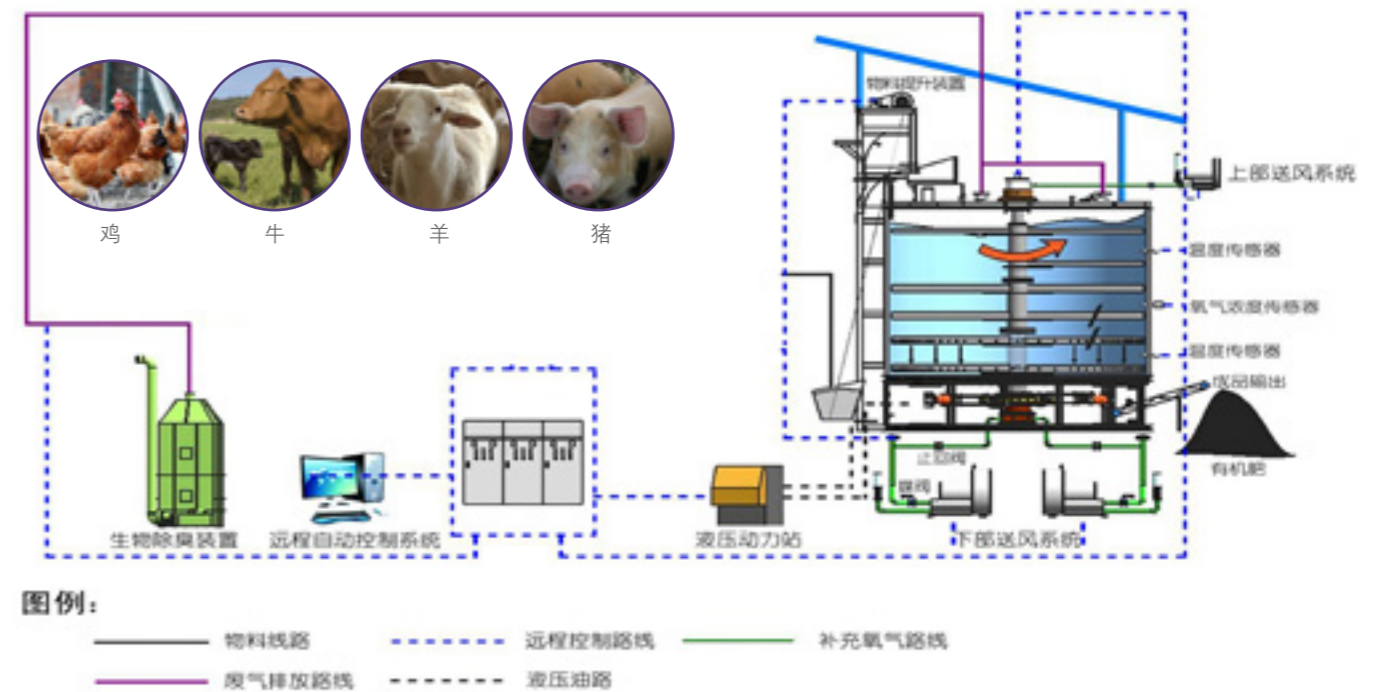
有机废弃物高温好氧发酵工艺流程图
